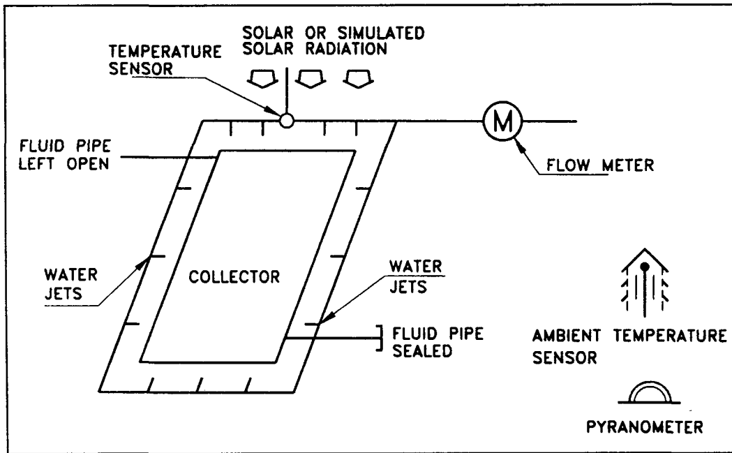
FIG. 2 EXTERNAL THERMAL TEST
