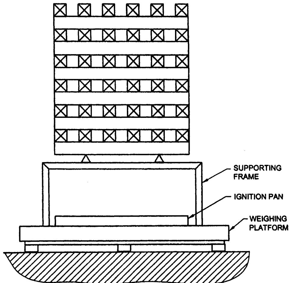
FIG. 2 CRIB FIRE
