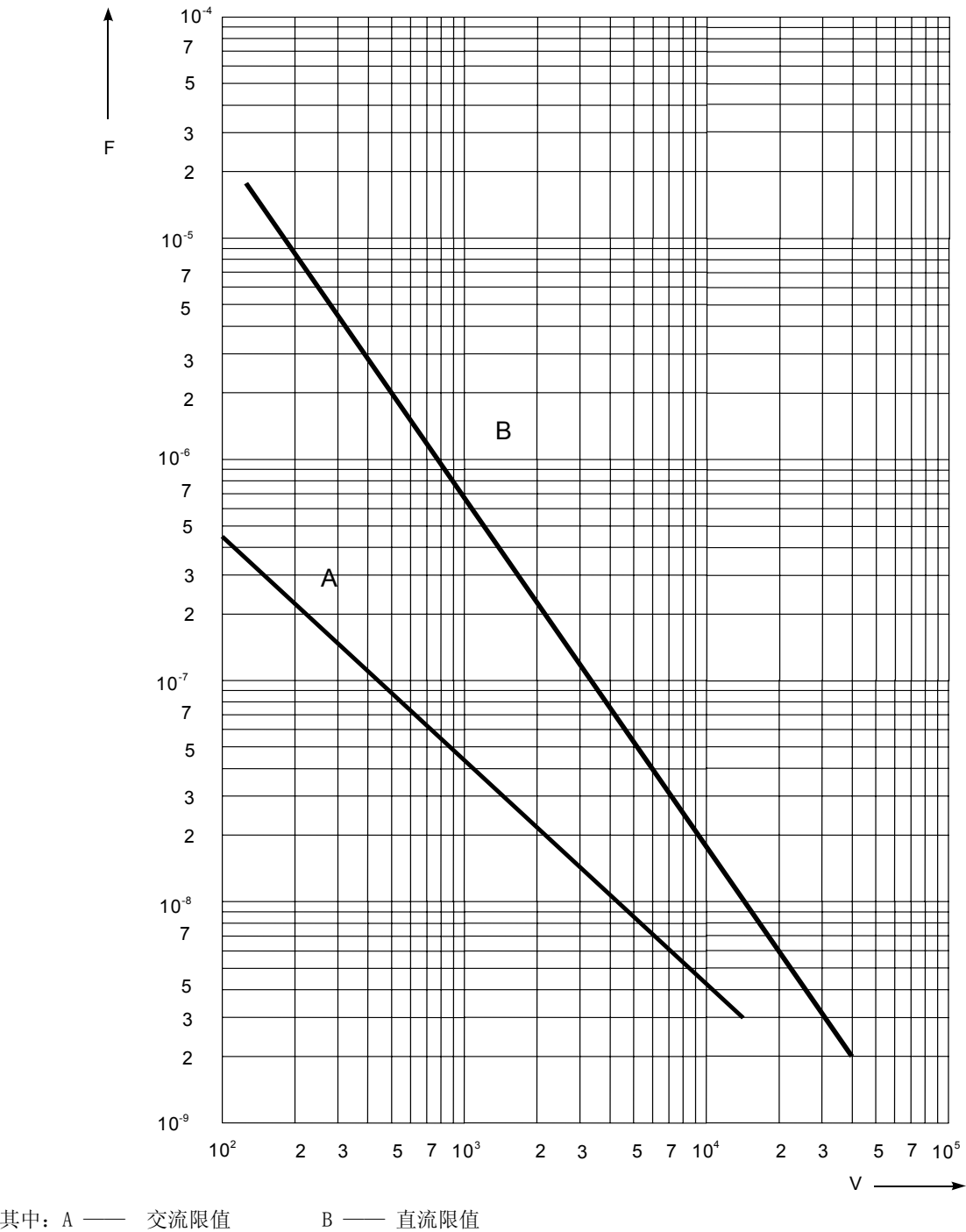
图1 正常条件和单一故障条件下充电电容量限值
