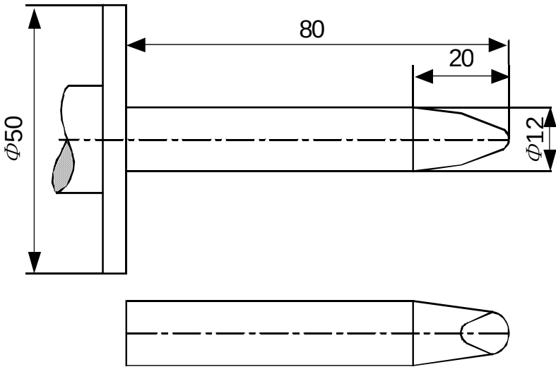
图 A. 1 刚性试验指（GB/T 16842 的试具 11）
