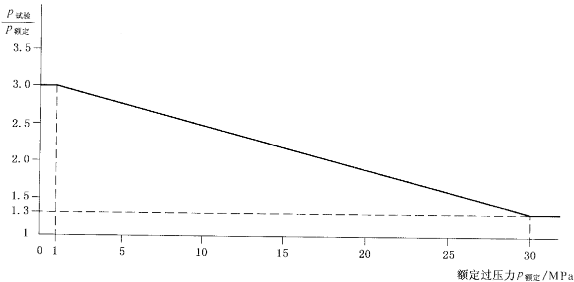
图2 液压试验的压力与额定最大工作压力之比
