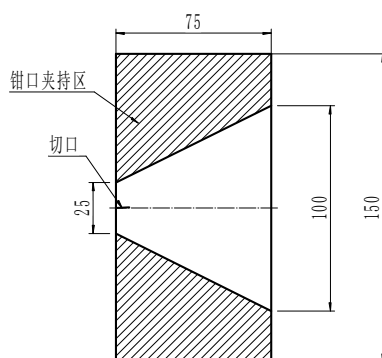
图1 梯形法撕裂强力试样夹持示意图
