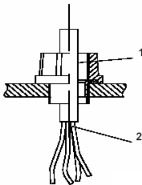
图 3b 导管引入方式
