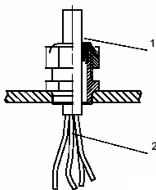
图 3a 电缆引入装置
