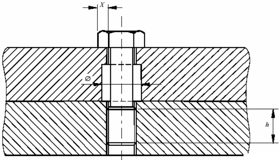
图1 螺纹紧固件的公差和间隙
