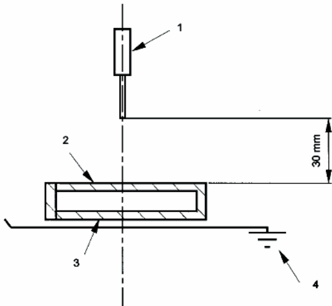
图7 用接地探针通过 0.1μF 电容给容器放电
