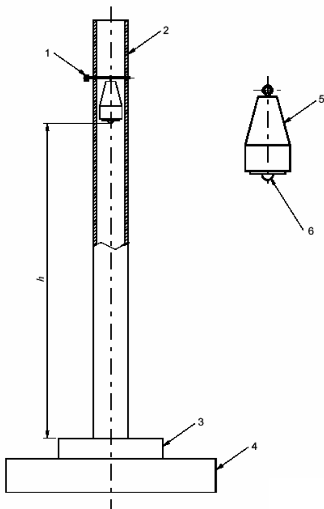
图 G.1 冲击试验装置示例
