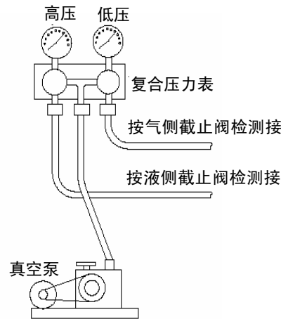
图 3 真空泵排空操作示意图
