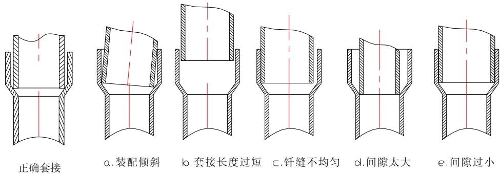
图 1 连接管正确套接方式
